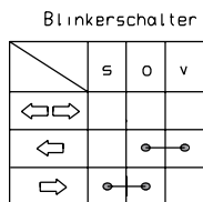
Kontaktbelegung - Lichtschalter (Typ CEV 9610)
