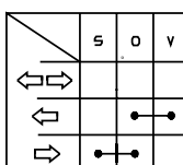
Blinkerschalter
