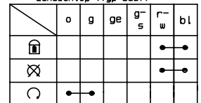
Zündschloß (Typ Zadi)
