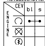
Zündschloß (Typ Zadi)
