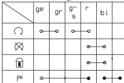
Zündschloß (Typ Zadi)
