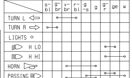
Kombischalter (Typ CEV 100826000)
